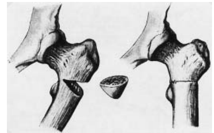
Abb. 7 „Keilförmige“ Osteotomie.
