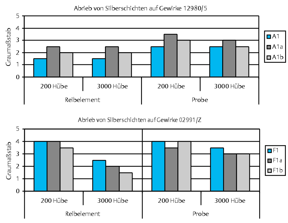
Abb. 6 Reibbeanspruchung mit Baumwoll-läppchen. Beurteilung des Reibelementes und der 3D-Gewirkeoberfläche mit Graumaßstab (200 und 3000 Reibtouren). Beurteilungskriterien: Note 5: kein Abrieb, keine erkennbare Beeinflussung der Reibstrecke. Note 1: großer Abrieb, Silberschicht befindet sich nicht mehr auf der Gewirkeoberfläche.
