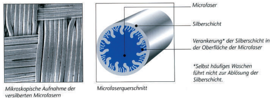
Abb. 4 Silberummantelte Polyamid-Mikrofasergarne; Quelle: Tex-A-Med GmbH.
