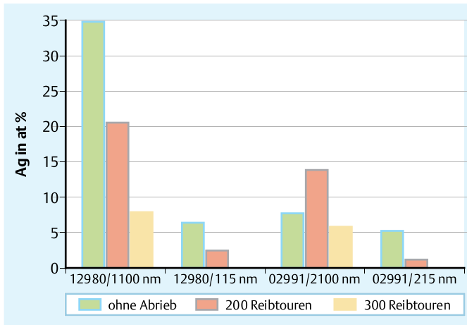
Abb. 8 Silberkonzentration an der Textiloberfläche nach Reibbeanspruchung.
