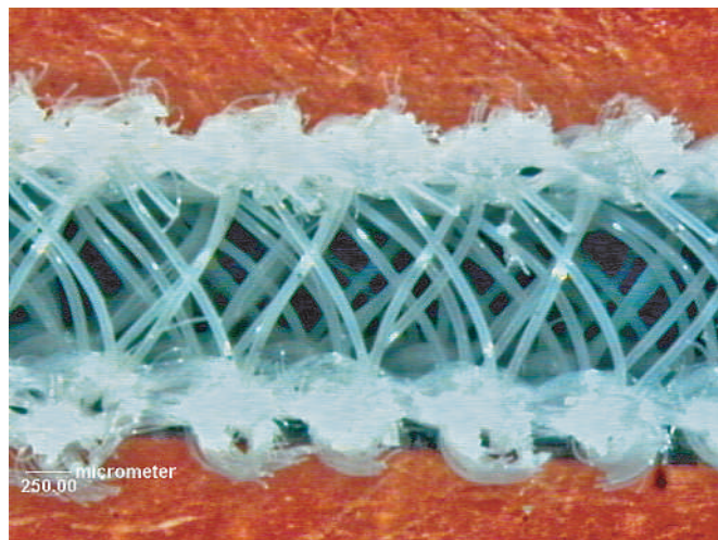
Abb. 1 Querschnitt durch ein 3D-Abstandsgewirke.
