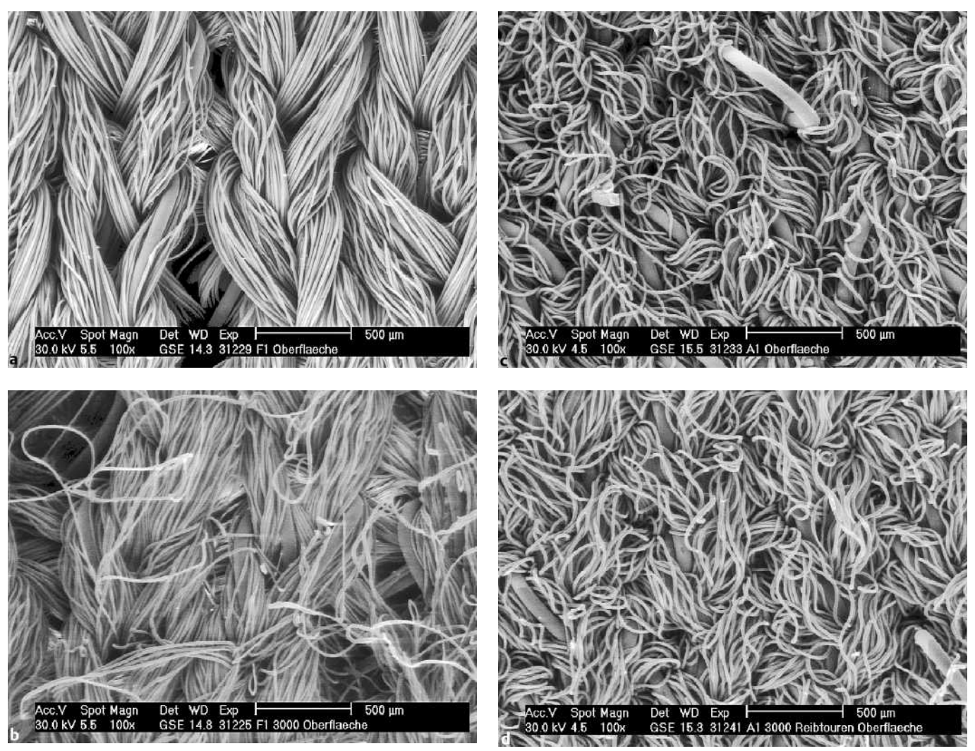
Abb. 7 a 3D-Gewirke 02991/Z, Oberfläche ohne Reibbeanspruchung. b Oberfläche nach 3000 Reibtouren. c 3D-Gewirke12980/5 Oberfläche ohne Reibbeanspruchung. d Oberfläche nach 3000 Reibtouren.
