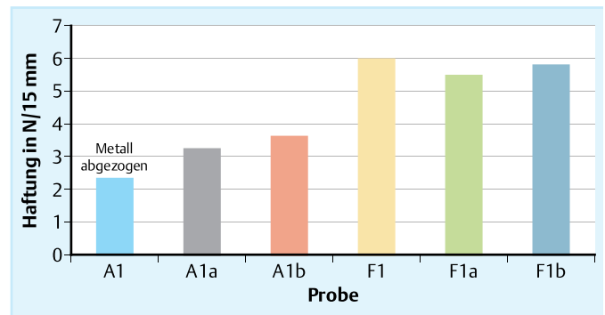
Abb. 5 Haftvermögen von Silberschichten auf unterschiedlichen Gewirkeoberflächen
