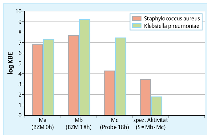
Abb. 3 Nachweis der antimikrobiellen Wirksamkeit von Silberionen nach der Testmethode JIL 1902.
