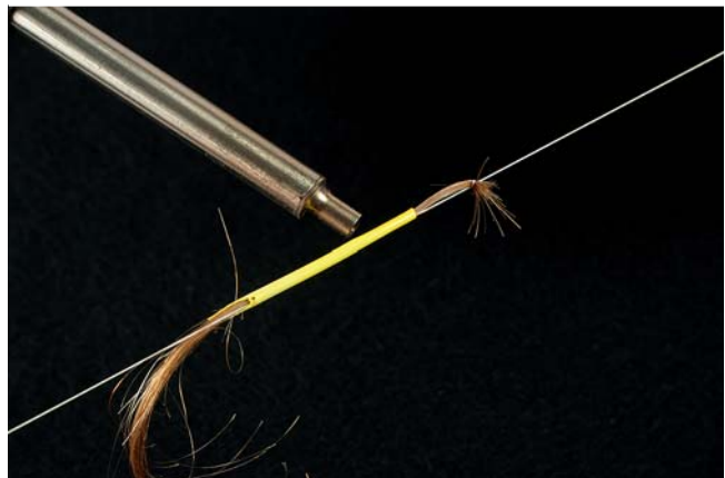
Abb. 4 Erwärmen des Schrumpfschlau- ches mit einer Heißluftpistole.
