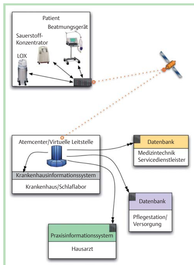
Abb. 1 Der Tele-Assistent für O 2 -Konzentratoren und LOX-Systeme in der Heimbeatmung [7]. Informationen von Geräten im Home-Care-Bereich werden an ein integriertes Funkmodul übermittelt, welches die Daten dann an die Empfangseinheit der Leitstelle sendet. Die Daten/Signale werden ausgewertet, gefiltert und intelligent zugeordnet.
