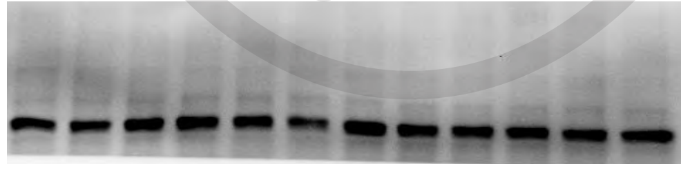
Total Akt
