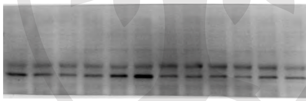
Total Akt
