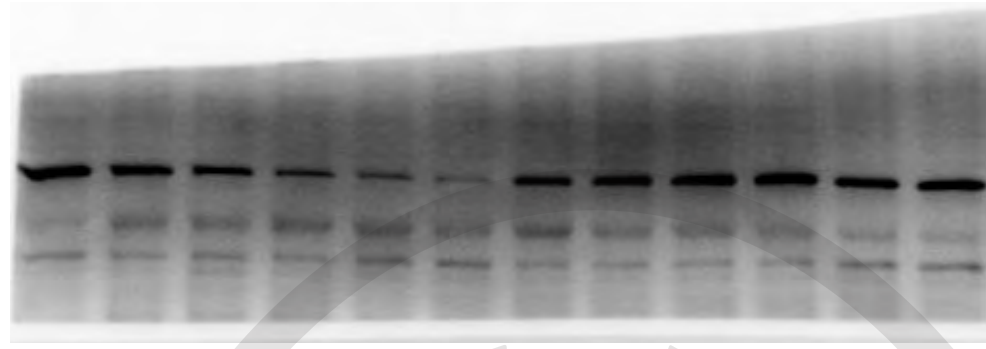
Akt S473
