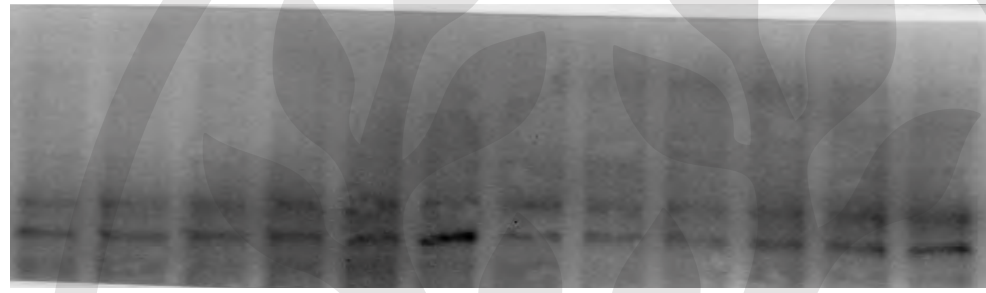
Akt S473
